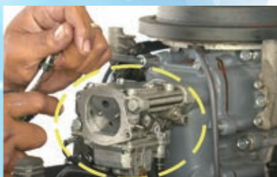
2ストローク船外機のキャブレター クランクシャフトケースに併設
